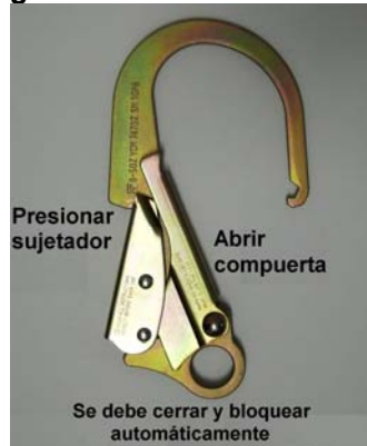
Fig. A-2 – Gancho de refuerzo
